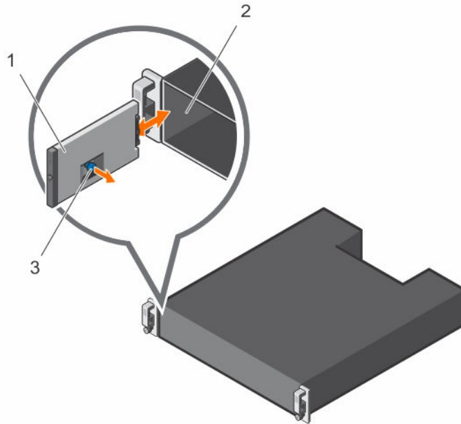
Abbildung 21. Bedienfeldplatine entfernen und installieren
