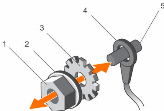
Abbildung 17. Schutzerdungskabel montieren und anschließen
