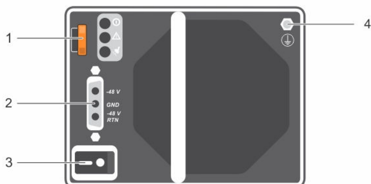
Abbildung 16. Rückseitenmerkmale eines Gleichstrom-Netzteilmoduls
