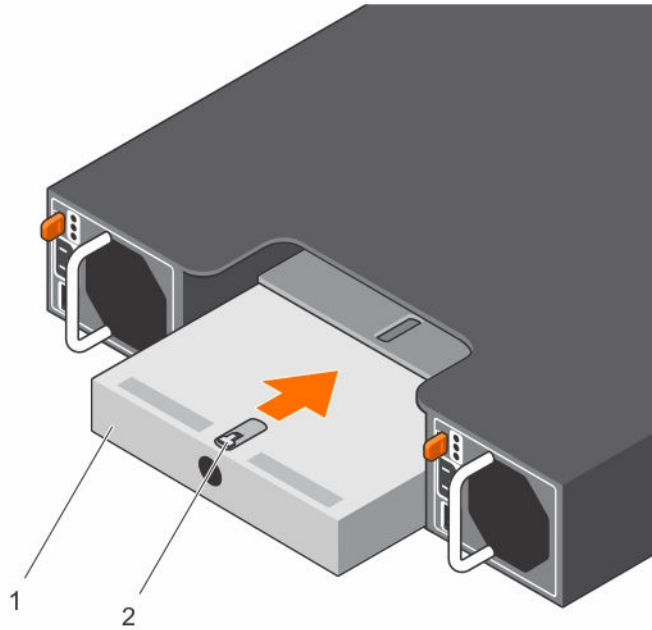
Abbildung 11. Entfernen und Installieren einer EMM-Platzhalterkarte
