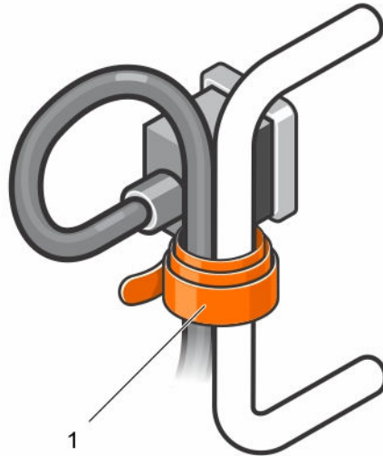
Abbildung 14. Befestigen der Stromkabel
